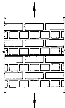
Рисунок 1 – Растяжение кладки по неперевязанному сечению
