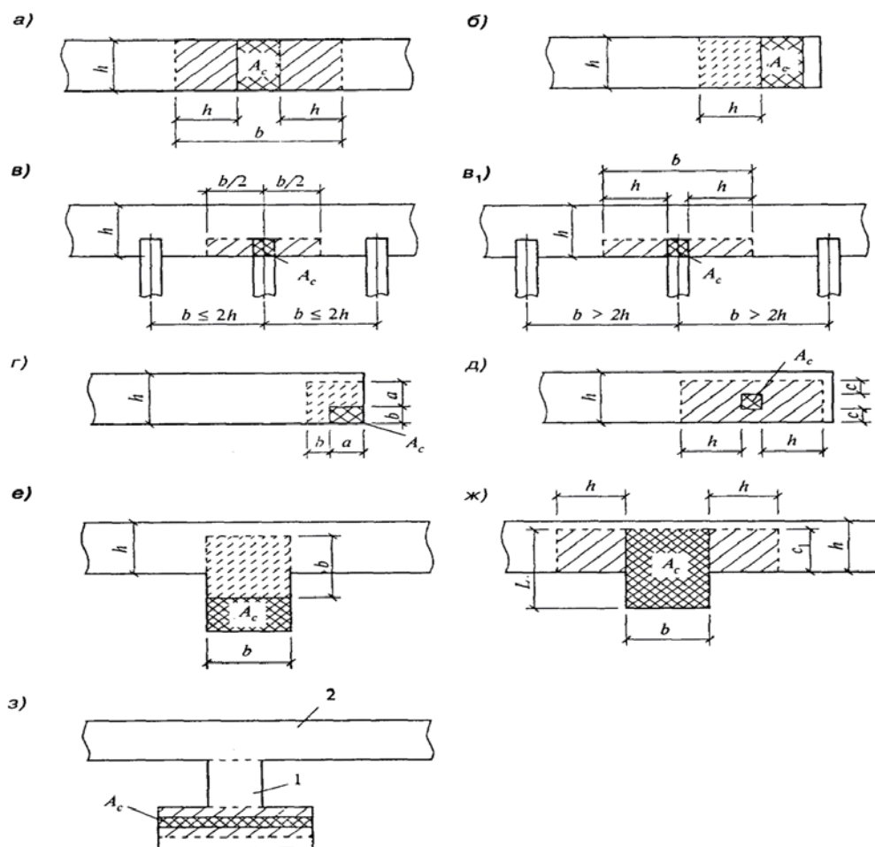
Рисунок 9 – Определение расчетных площадей сечений при смятии (местном сжатии)
