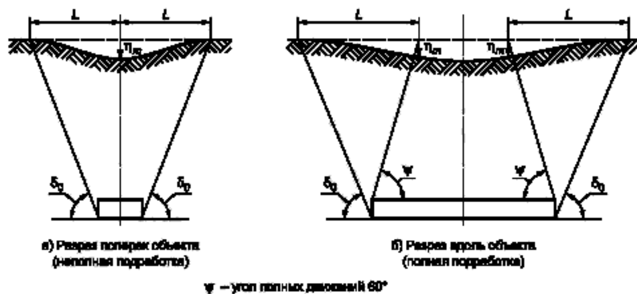
Рисунок Р.1 — Основные параметры мульты сдвижения
